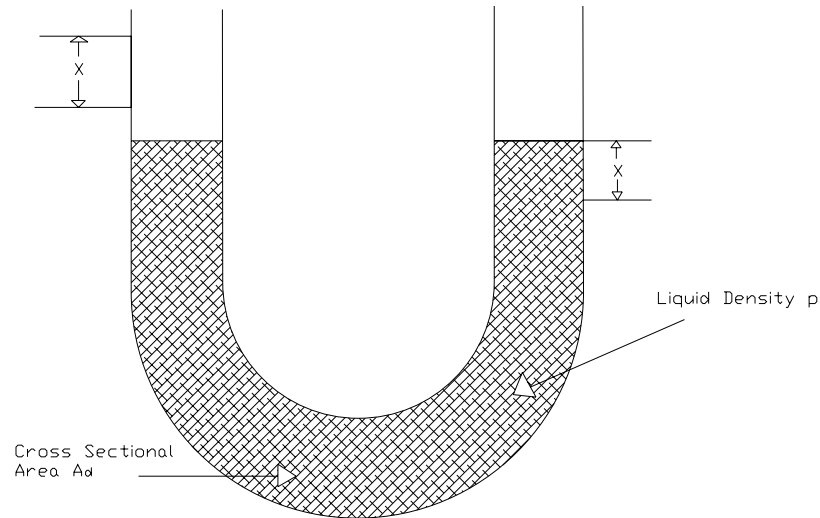
Fig.2.3.1 Simple Displacer U-Tube
